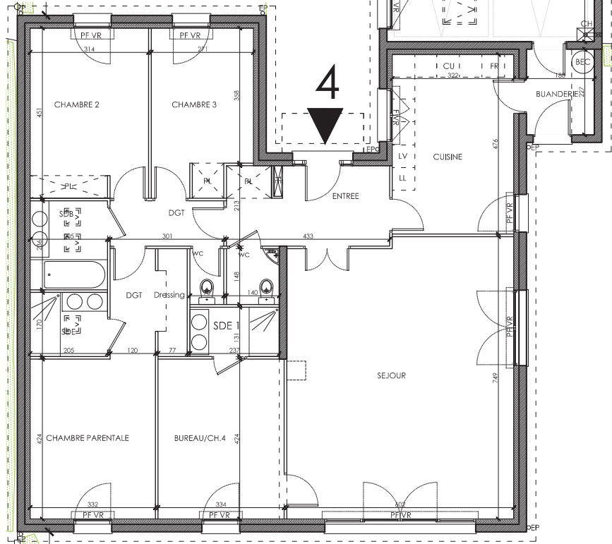
PLAN RDC
